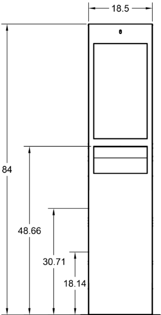
Wellness Kiosk - 32"
