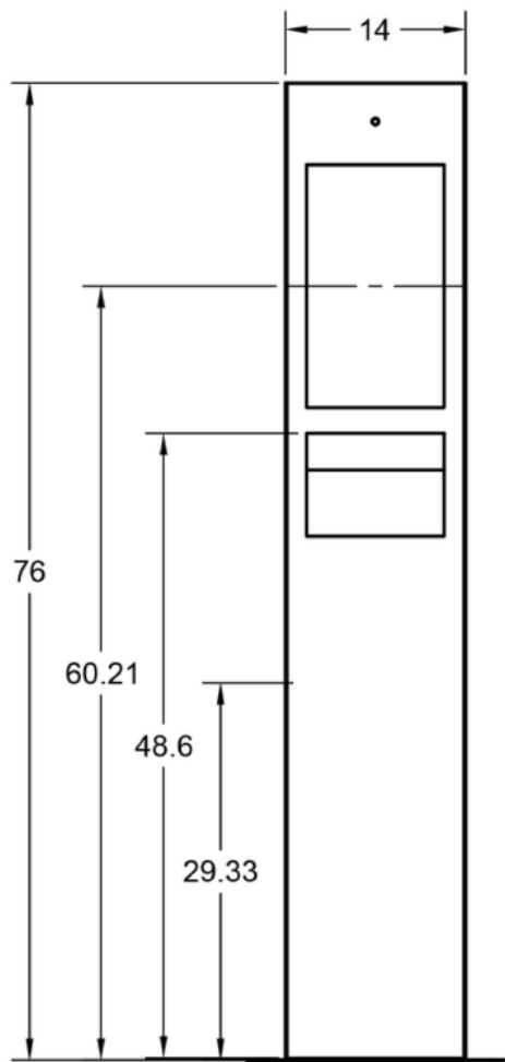
Wellness Kiosk - 22"
